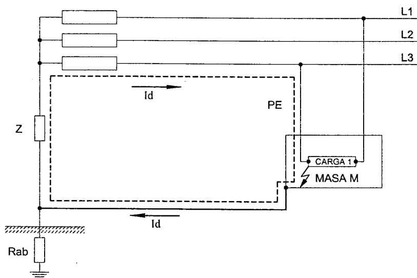
Fig. 771-H.A Esquema IT en el que el punto neutro está conectado a tierra a través de una impedancia Z y en el que los electrodos de tierra de la alimentación ( R_b ) y de las masas eléctricas de la instalación ( R_a ) están unificados en uno ( R_{ab} )
