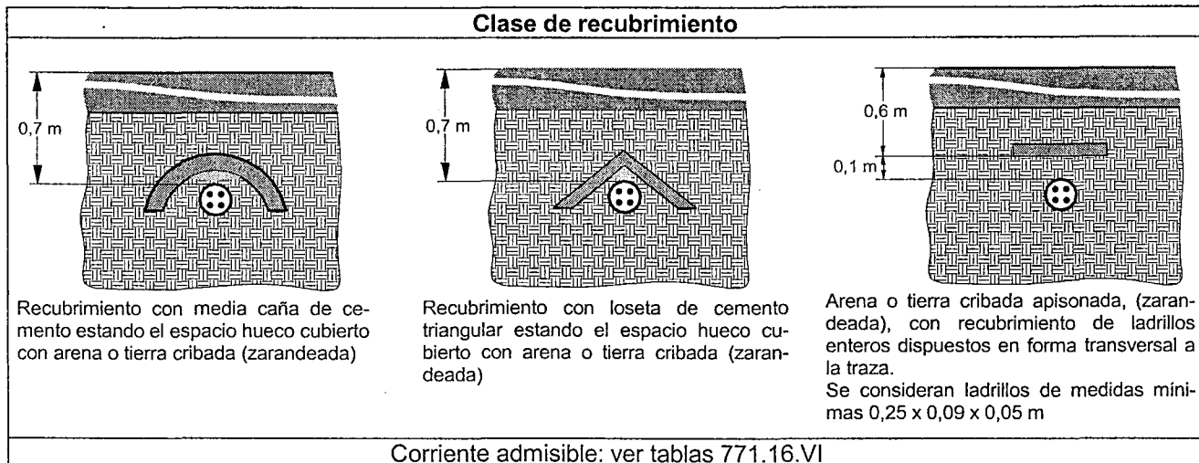
Figura 771.12.H – Protecciones contra el deterioro mecánico
