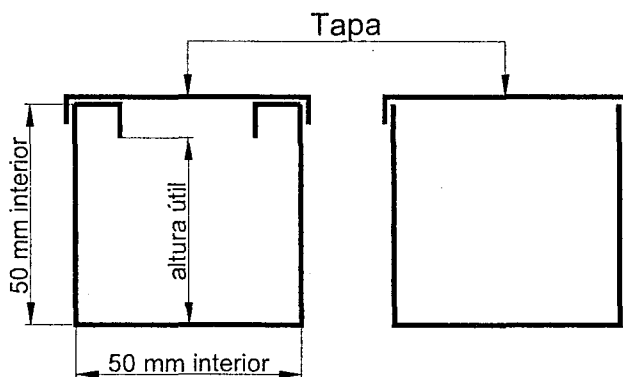
Figura 771.12.A – Perfil C típico (perfil registrable)
