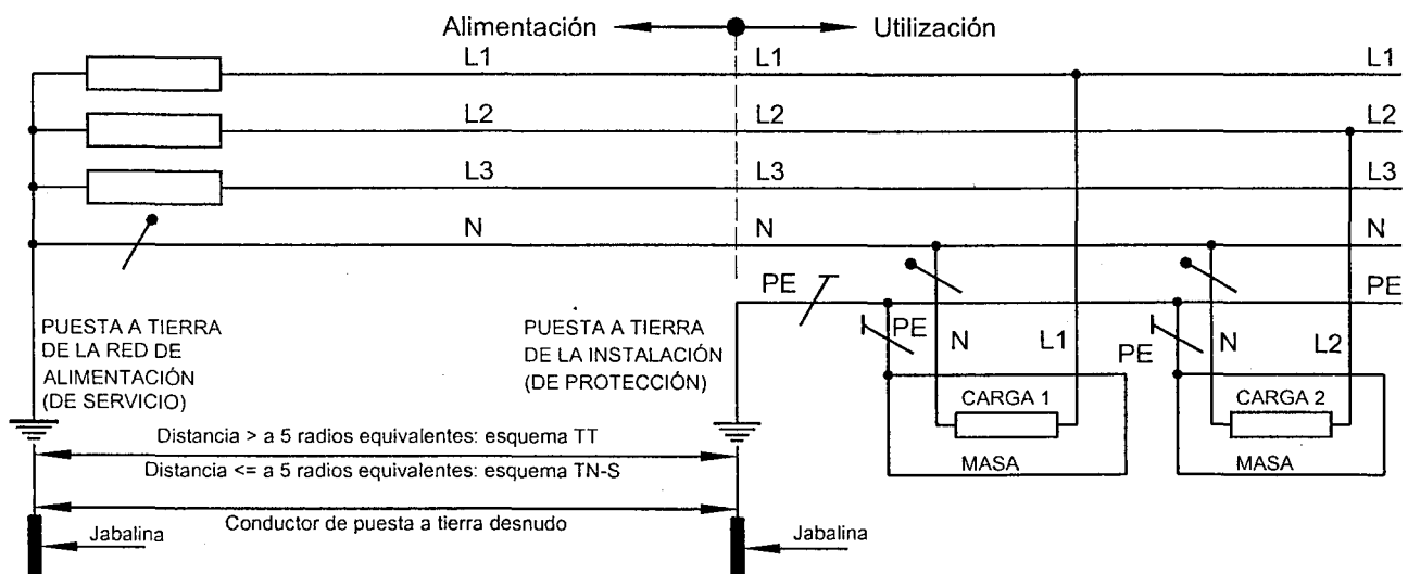
Figura 771.5.A – Separación entre sistemas de puesta a tierra (esquema 1)
