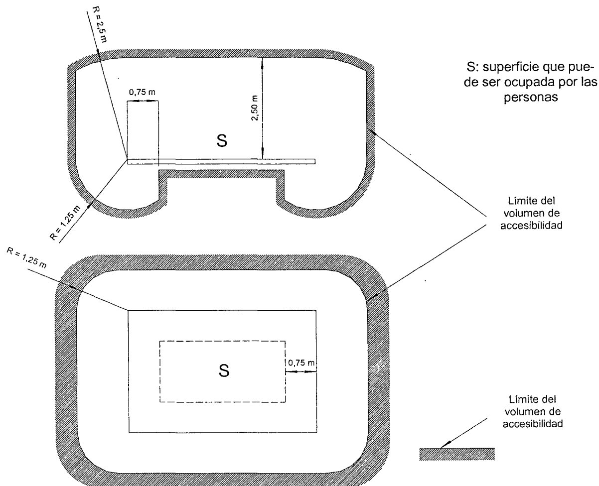
Figura 771.18.A – Zonas de accesibilidad
