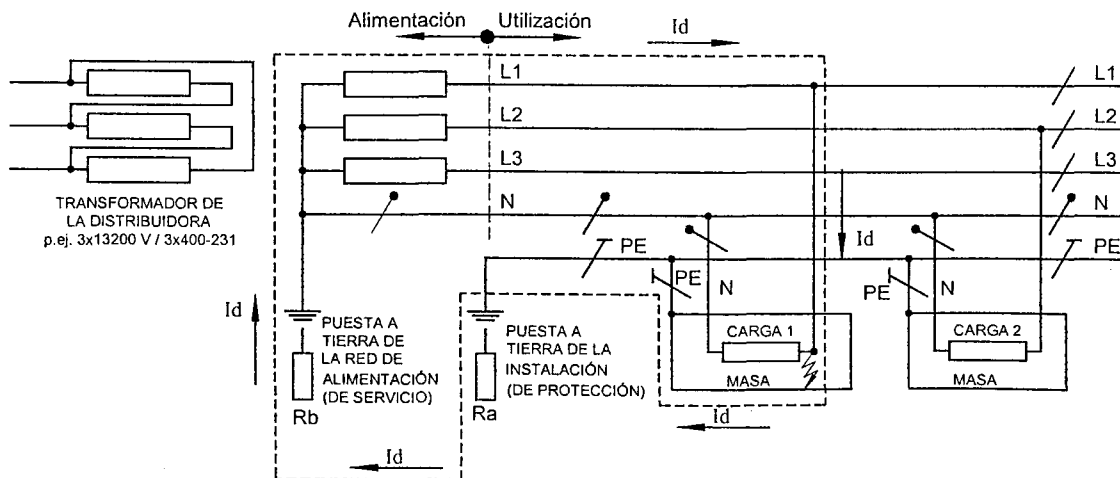
Figura 771.18.B – Lazo de falla esquema TT
