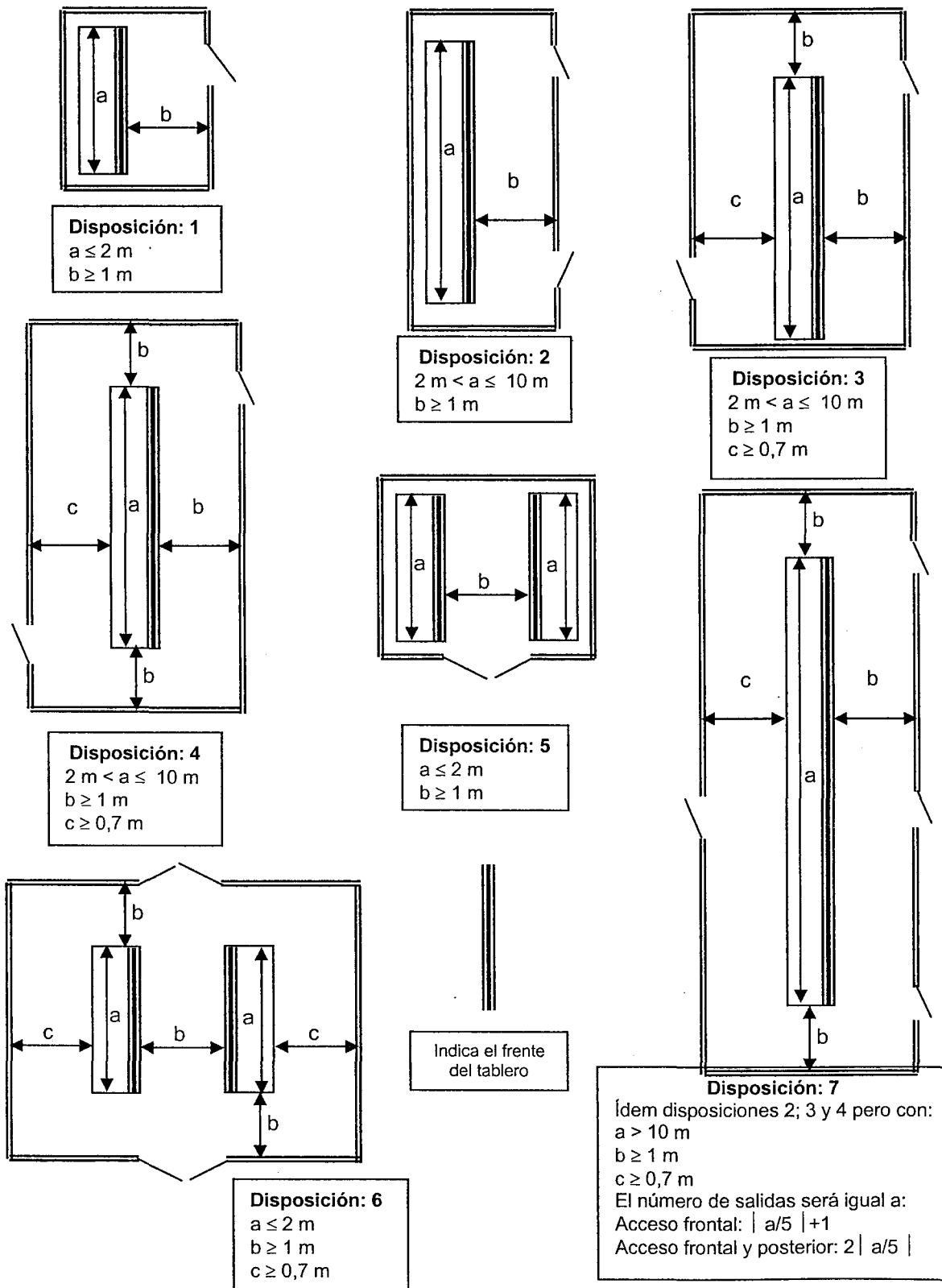
Figura 771.20.A- Disposición de tableros ubicados sobre el solado. (No se aplica a tableros embutidos)
