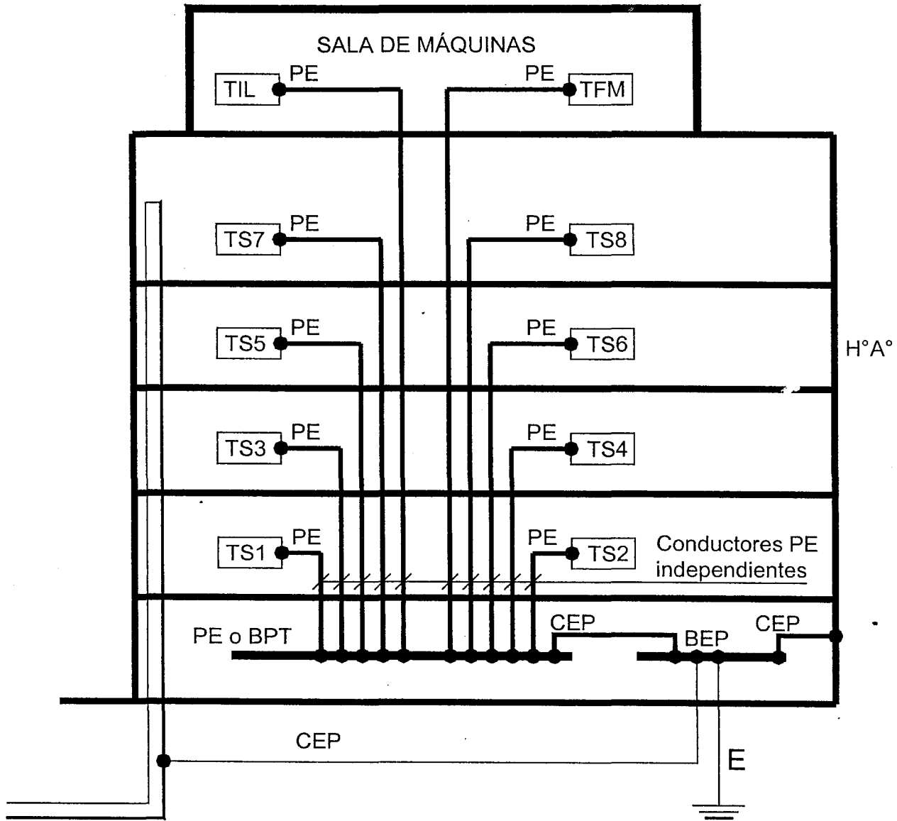
Figura 771.12.B - Ejemplo de inmueble con varios usuarios (conductores PE independientes)
