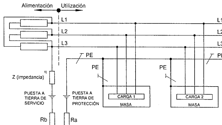
Figura 771.3.G - Esquema IT con neutro distribuido
