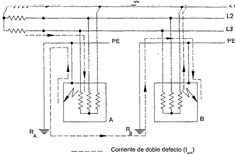
Fig. 771-H.B Corriente de doble defecto en el esquema IT cuando las masas no están conectadas a la misma toma de tierra. Este esquema no depende de la situación de la alimentación en relación con la tierra (aislada o conectada a tierra por una impedancia). Ver 413.1.5.5 a) donde se indican los requerimientos del esquema TT
