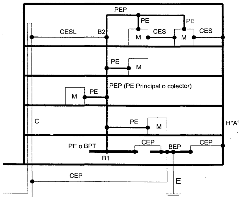
Figura 771.18.C – Ejemplo de equipotencialización
