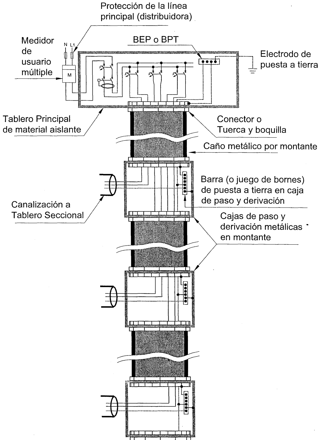
Figura 771.12.F - Ejemplo de equipotencialización de inmueble con un solo usuario
