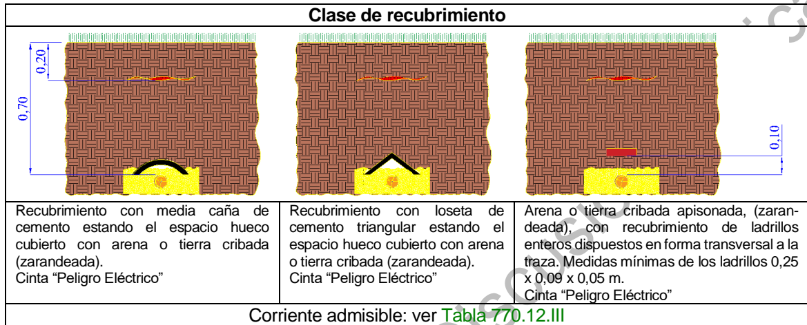
Figura 770.10.A - Protecciones contra el deterioro mecánico
