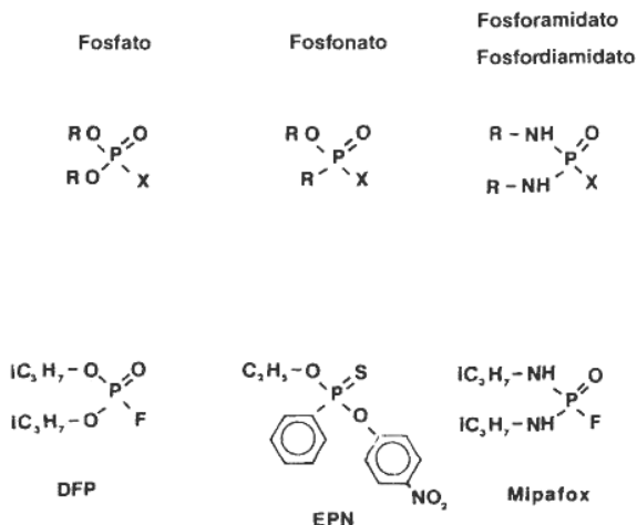
Fig. 22-2. Las estructuras básicas y la nomenclatura de los ésteres organofosforados, con ejemplos, capaces de producir neurotoxicidad tardía inducida por organofosfato (OPIDN).
