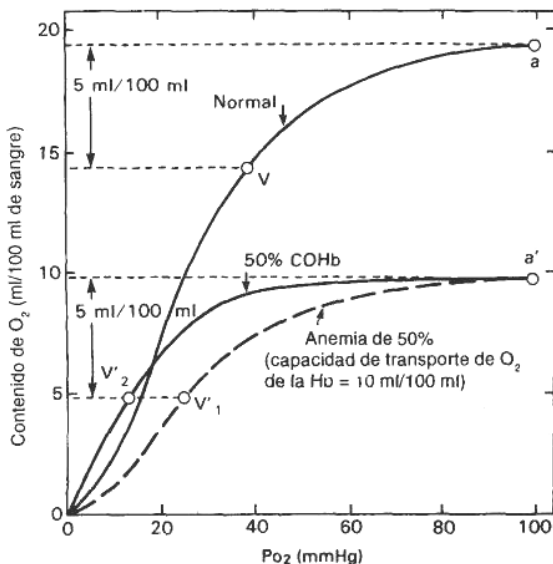
Fig. 11-3. Curva normal de disociación de la oxihemoglobina, y curvas para el caso de una anemia de 50% y el caso de una carboxihemoglobinemía de 50%. La liberación de 25% del volumen total de oxígeno de sangre arterial por completo oxigenada (5 ml/100 ml de sangre) requiere una disminución de la P_{O_2} de alrededor de 60 mm Hg (desde el punto a hasta el punto V en la curva normal). La liberación de un volumen comparable de oxígeno en el caso de una anemia de 50% exige un decremento de la P_{O_2} de más de 75 mm Hg (desde el punto a' hasta el punto V 1 ), pero se necesita una disminución aún mayor de la P_{O_2} para liberar el mismo volumen de oxígeno en el caso de la curva alterada por la presencia de carboxihemoglobina (desde el punto a' hasta el punto V 2 ).
