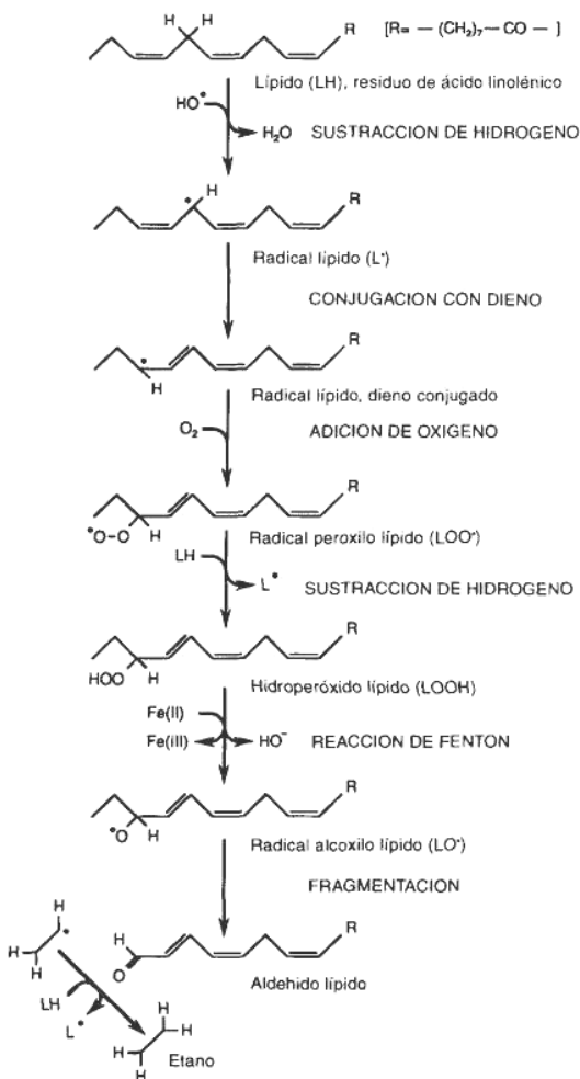
Fig. 3-2. Peroxidación de lípidos comenzada por el radical hidroxilo (HCT). Muchos de los productos, como los radicales y los aldehídos a, P-insaturados, son reactivos, en tanto otros, como el etano, son no reactivos, pero son indicadores de peroxidación de lípidos.
