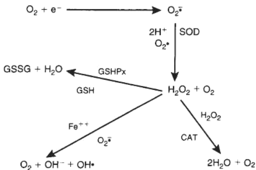
Fig. 17-3. Formación e inactivación de especies de oxígeno reactivas. La reducción de oxígeno de electrón único produce la formación de radical anión superóxido ( \text{O}_2^{\cdot -} ), que se mantiene a concentraciones intracelulares bajas por medio de dismutación espontánea o rompimiento catalítico por la enzima superóxido dismutasa (SOD) para formar peróxido de hidrógeno ( \text{H}_2\text{O}_2 ). Pueden ocurrir tres fenómenos posibles con el \text{H}_2\text{O}_2 : 1) en presencia de \text{O}_2^{\cdot -} o metales de transición, como el hierro y el cobre, se reduce hacia el radical hidroxilo ( \text{OH}^{\cdot} ); 2) puede catalizarse por la catalasa (CAT) para formar agua y oxígeno, y 3) puede detoxificarse mediante la glutatión peroxidasa (GSHPx) en presencia de glutatión (GSH) para formar agua y glutatión oxidado (GSSG).
