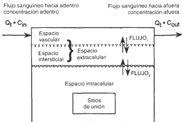
Fig. 7-4. Representación esquemática de un compartimento unido en un modelo fisiológico. Véase el significado de las siglas en el texto.
