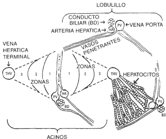
Fig. 13-1. Esquema de las unidades operativas hepáticas: lobulillo clásico y acino. El lobulillo está centrado en la vena hepática terminal (vena central), donde la sangre drena hacia afuera del lobulillo. El acino tiene como su base los vasos penetrantes, por medio de los cuales la sangre aportada por la vena porta y la arteria hepática fluye por el acino hasta más allá de los cordones de hepatocitos. Las zonas 1, 2 y 3 del acino representan regiones metabólicas cada vez más distantes del aporte sanguíneo.
