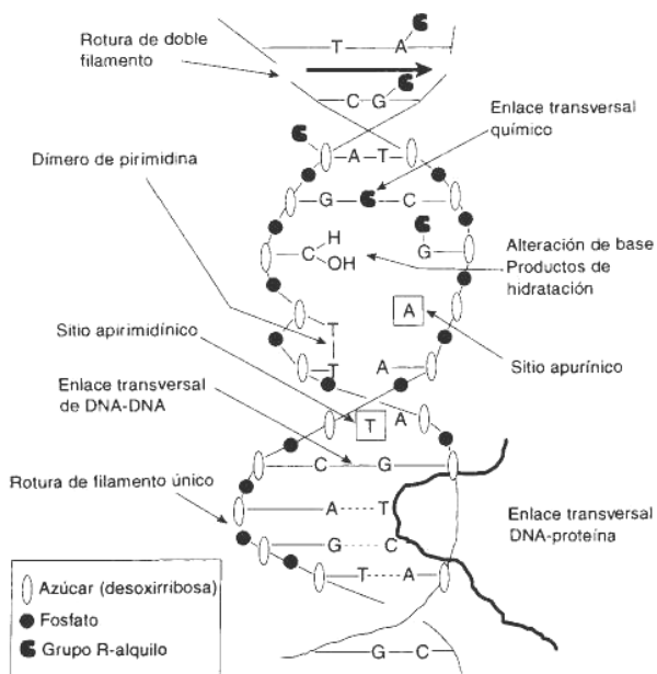
Fig. 8-1. Representación esquemática de lesiones del DNA inducidas por sustancias químicas y radiación.
